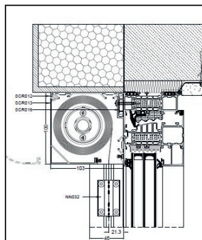
Ablak tokra szerelés (A)
