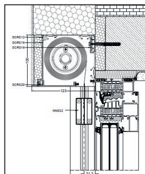
Áthidalóra szerelés, ha az áthidalón már van szigetelés (A)
