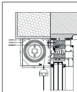
Ablak tokra szerelés (B)
