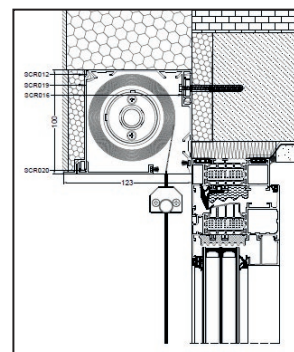
Áthidalóra szerelés, ha az áthidalón már van szigetelés (B)
