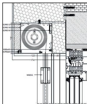
Áthidalóra szerelés, előtte és mögötte extra szigeteléssel
