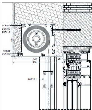
Áthidalóra szerelés, előtte és mögötte szigetelőlemezzel
